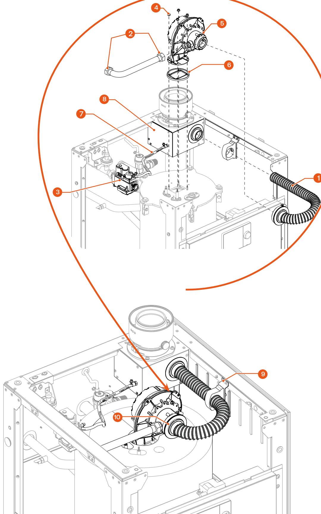
Rys. 24. Demontaż i montaż zespołu wentylatora i mieszacza gazu i powietrza
