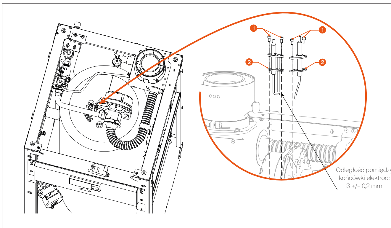
Rys. 23. Demontaż i montaż elektrod
