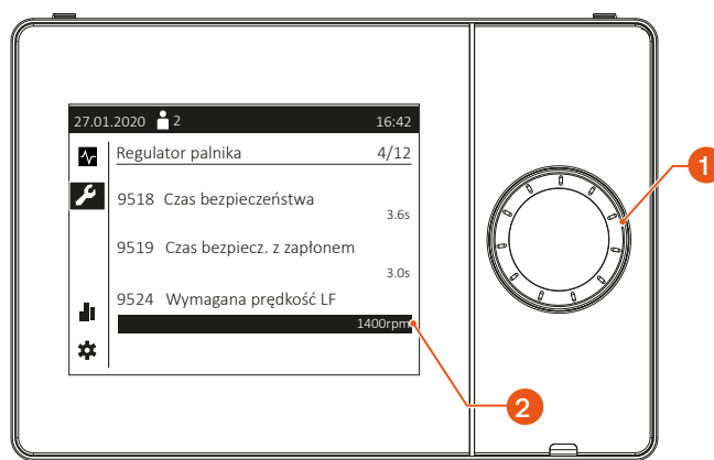
Rys. 18. Regulacja prędkości pracy wentylatora — widok wyświetlacza
